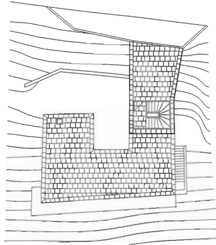
Eingangsgeschoss
