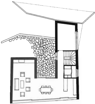
Wohngeschoss
